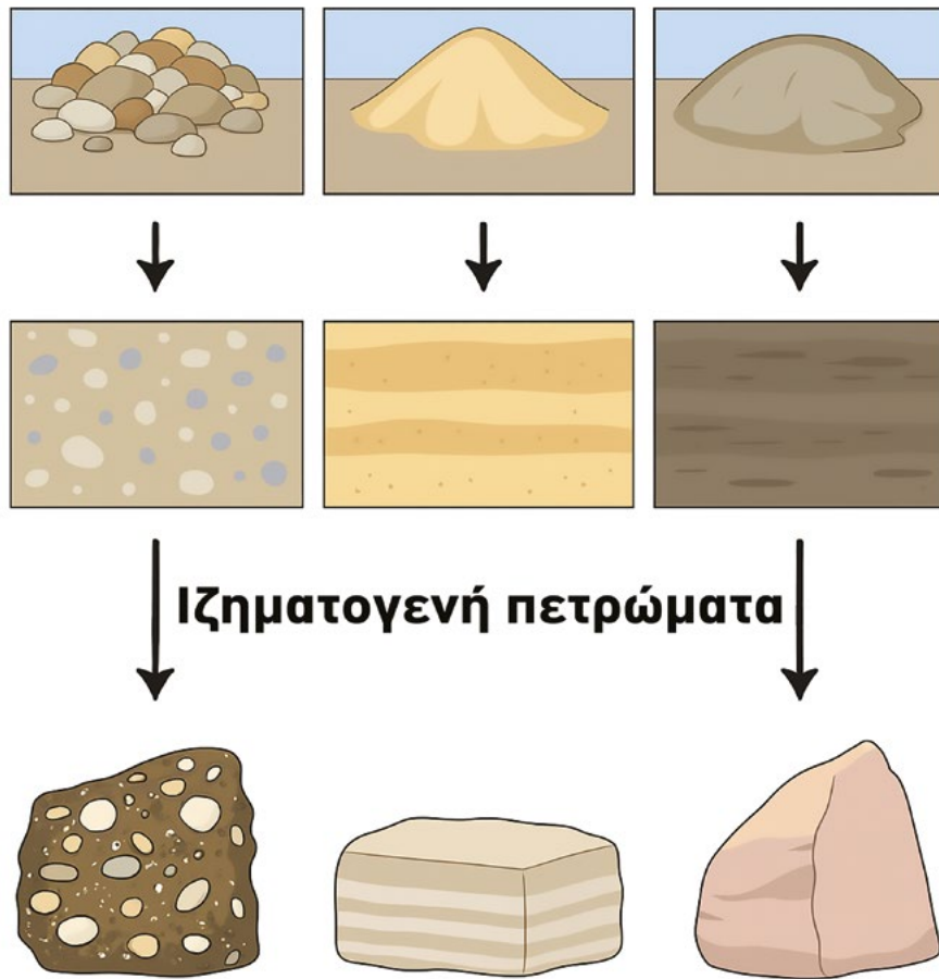
Εικ. 14.1. Ιζήματα και Ιζηματογενή πετρώματα
