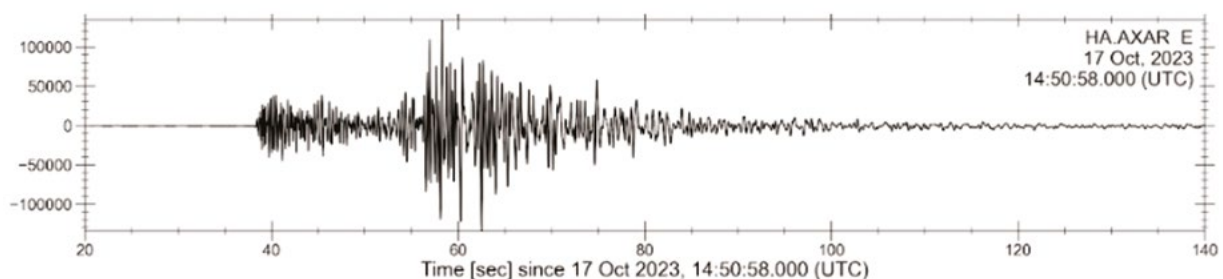
Εικ.10.3. Σεισμογράμμα
